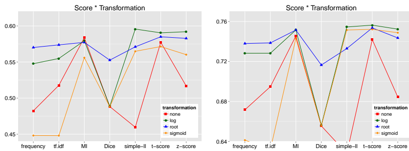
Almuhareb & Poesio
