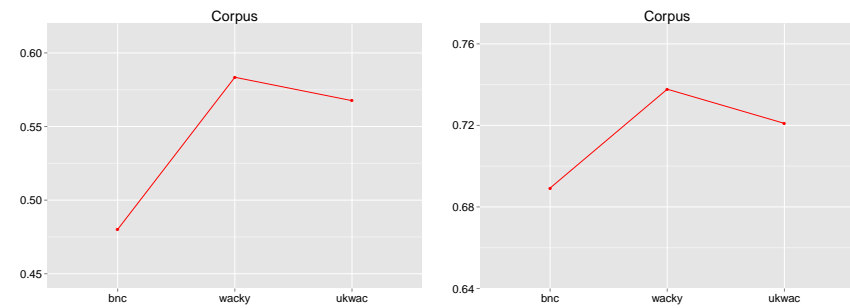
Almuhareb & Poesio
